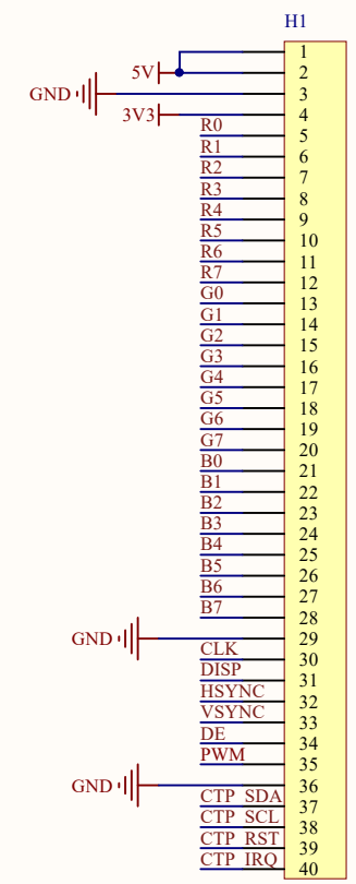
RGB Cable Interface
