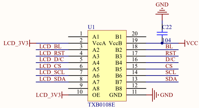
Level shift
