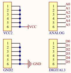
Analog_In
