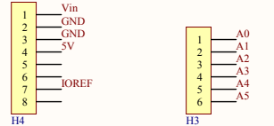
Main_Board_In
